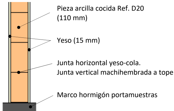
Esquema de muestra ensayada (B2021-151-M837)
